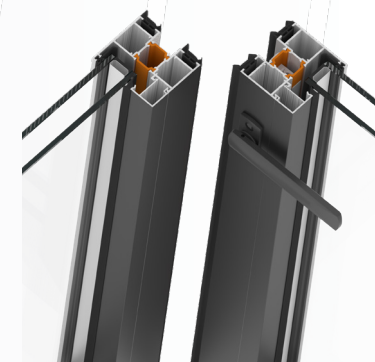
Деталь наружной складной двери показана выше.
