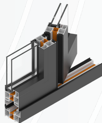
Соединение створка-к-створке SKYFOLD выполняется так, как показано выше.
