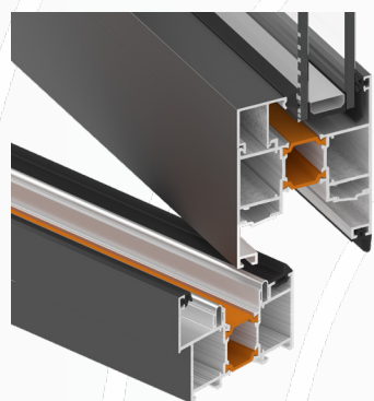
Деталь нижней рамы и створки крупным планом.
