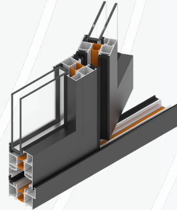
SKYFOLD kanat-kanat bağlantısı yukarıda gösterildiği şekilde yapılmaktadır.
