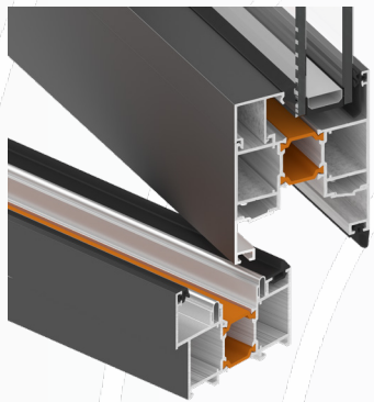
Alt kasa ve kanat detayı yakın planda.
