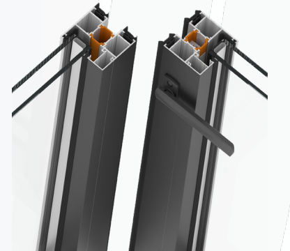
Dış katlanır kapı detayı yukarıda gösterilmiştir.
