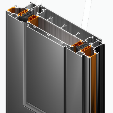
Ventsash pencere-kapı sistemi bağlantı detayı, kapalı pozisyonda.
